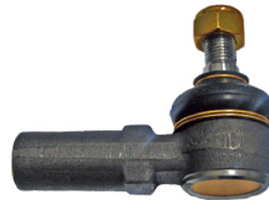
Ref.: 4014 EXTREMO L=80 MM. (RH.14x1.50)
